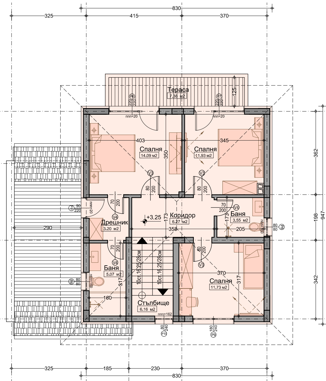
РАЗПРЕДЕЛЕНИЕ ВТОРИ ЕТАЖ М 1:100 ЗАСТРОЕНА ПЛОЩ: 87.28м 2
